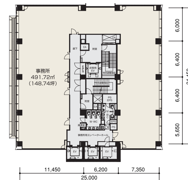
10階平面図
