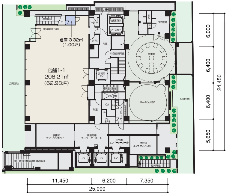
1階平面図
