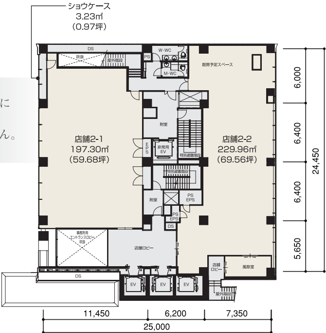
2階平面図
